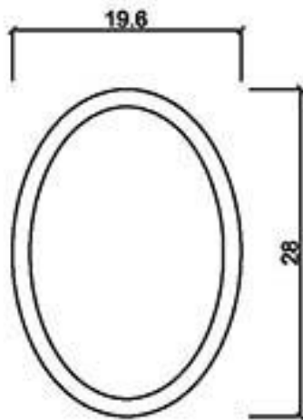
型號 MW-2030
