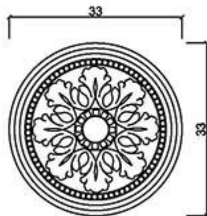
型號 MW-0533
