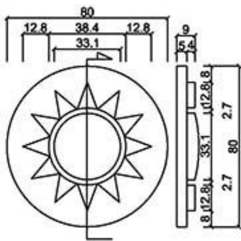
型號 MW-0980
