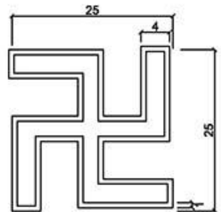
型號 MW-2040
